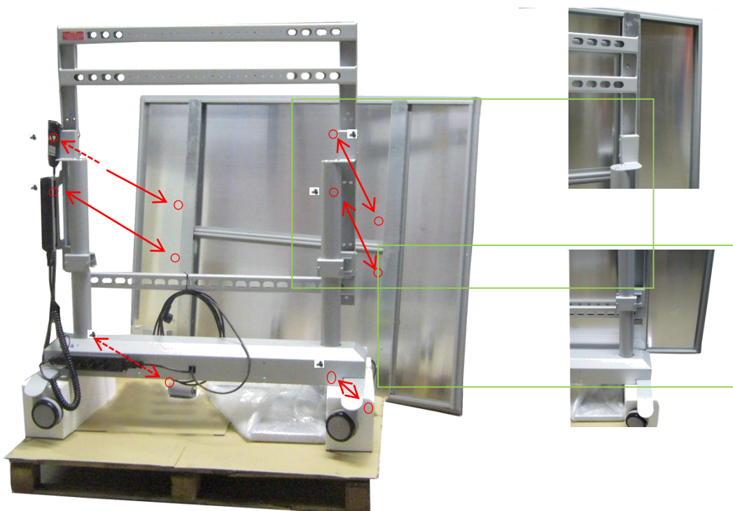
Boardadapter verschraubt mit Board
